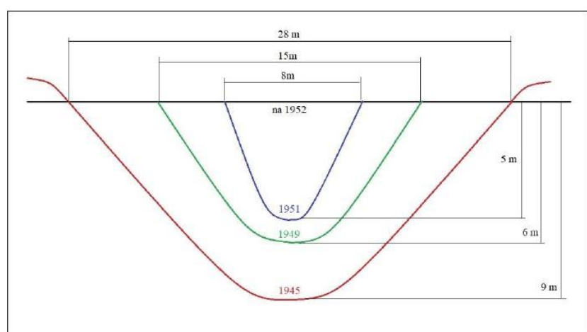
Fig. 86. Evolutie van de vorm van de krater van de NA197 op basis van waarnemingen. De maten zijn indicatief. Tekening: Alfons Bruekers.
